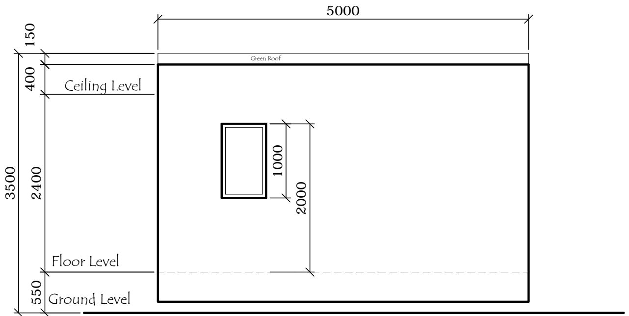
RIGHT ELEVATION
