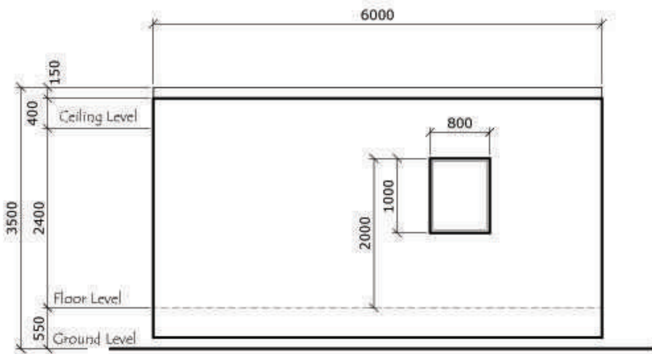
Right Side Elevation SCALE: 1:50 M
