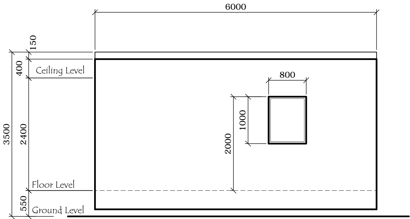
Right Side Elevation SCALE: 1: 50 M
